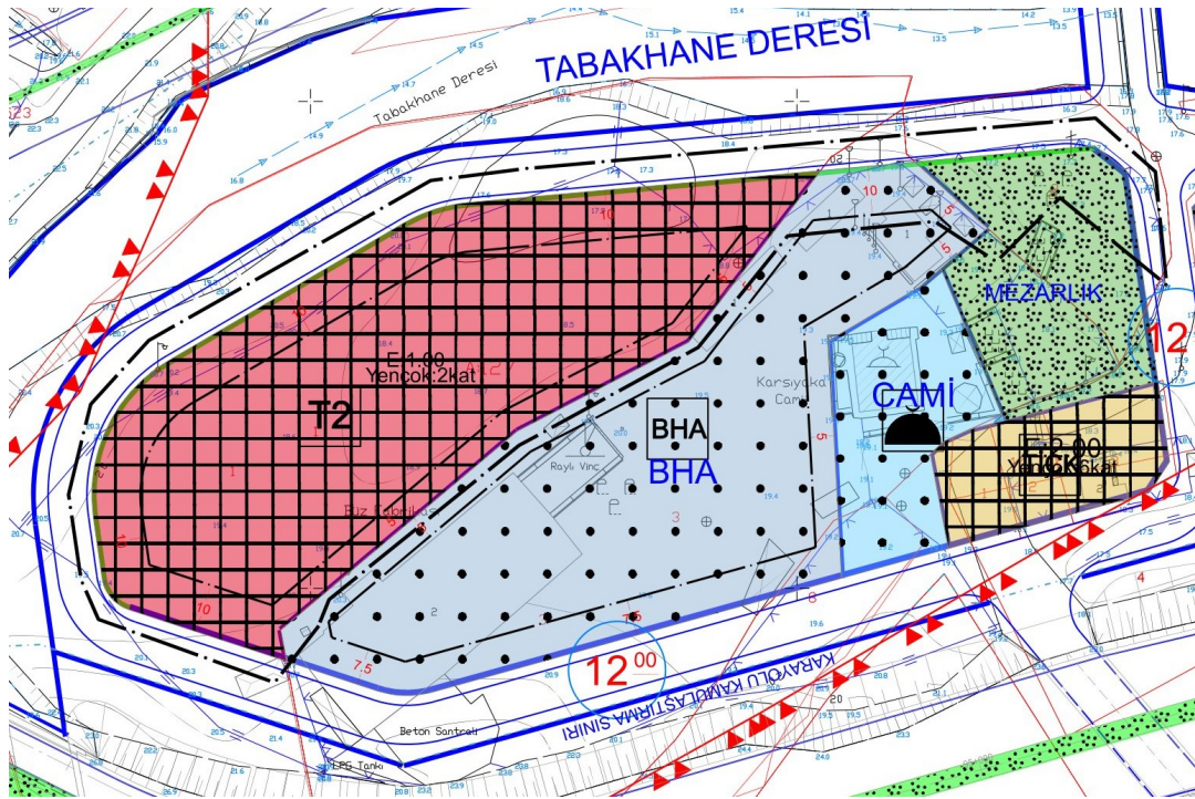
PLAN DEĞİŞİKLİĞİ
