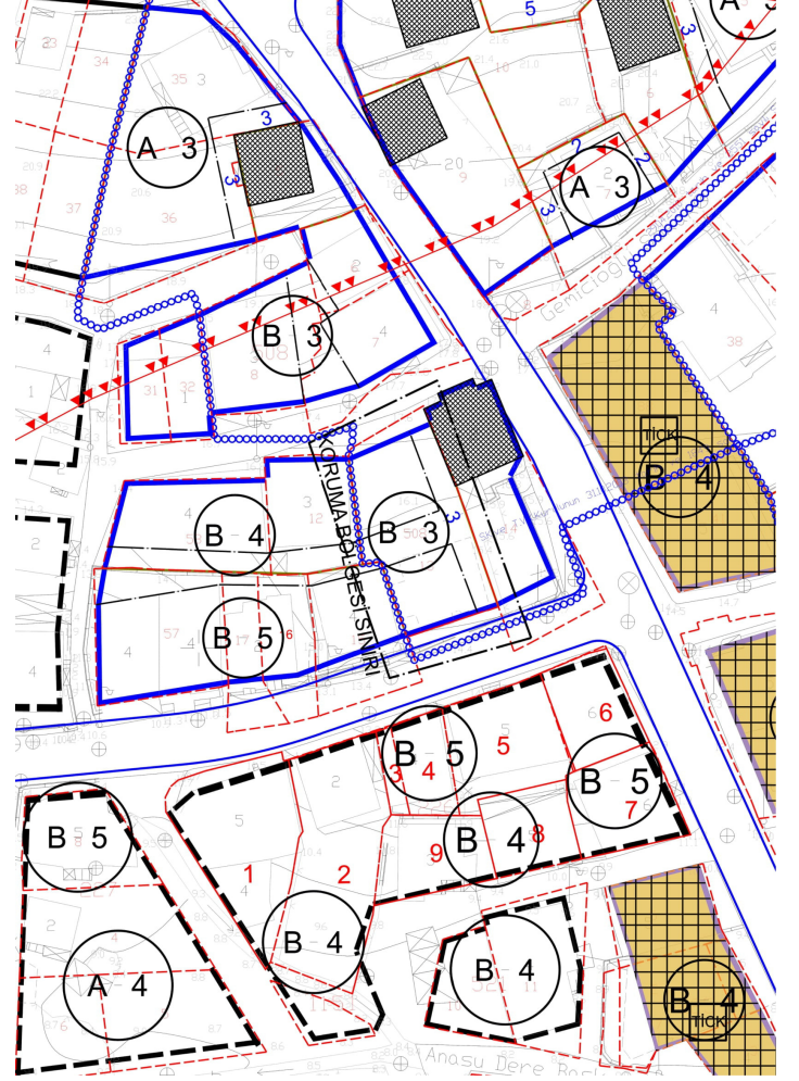
PLAN DEĞİŞİKLİĞİ
